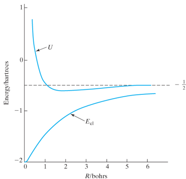
图 13.4: \text{H}_2^+ 基态电子能级中存在 ( U ) 和不存在 ( E_{\text{el}} ) 核间排斥势的电子能量。
