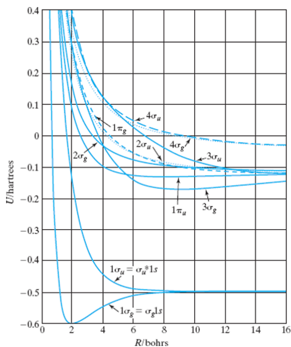
几个 \text{H}_2^+ 电子态的 U(R) 曲线。虚线用于帮助区分间隔较近的能级。在本图的尺度上无法观察到第一激发电子能级曲线在 12.5 bohrs 处的一个微小谷值，其势阱深度为 0.00006 hartrees。
